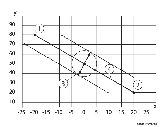
Bild 4 Außentemperaturgeführte Heizkurve
