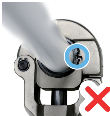
Spalt vorhanden
