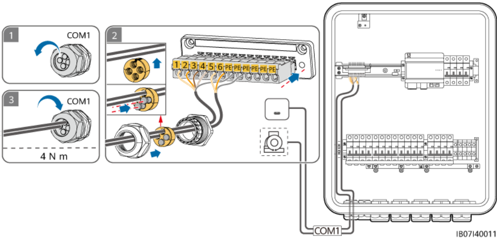
Abbildung 5-27 Anschluss der SmartGuard-Signalkabel (das gestrichelte Kästchen zeigt eine optionale Komponente an)
