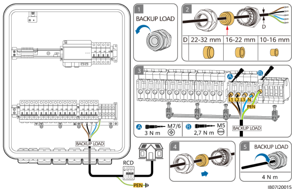
Abbildung 5-18 Anschließen des Ausgangsstromkabels der Backup-Last vom SmartGuard-63A-T0 (TN-S/TN-C-S/TT-System)
