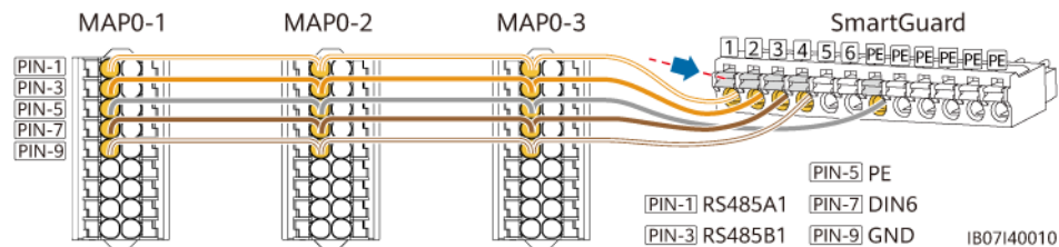
Abbildung 5-26 Parallelschaltung von Signalkabeln (am Beispiel von drei parallel geschalteten Wechselrichtern)
