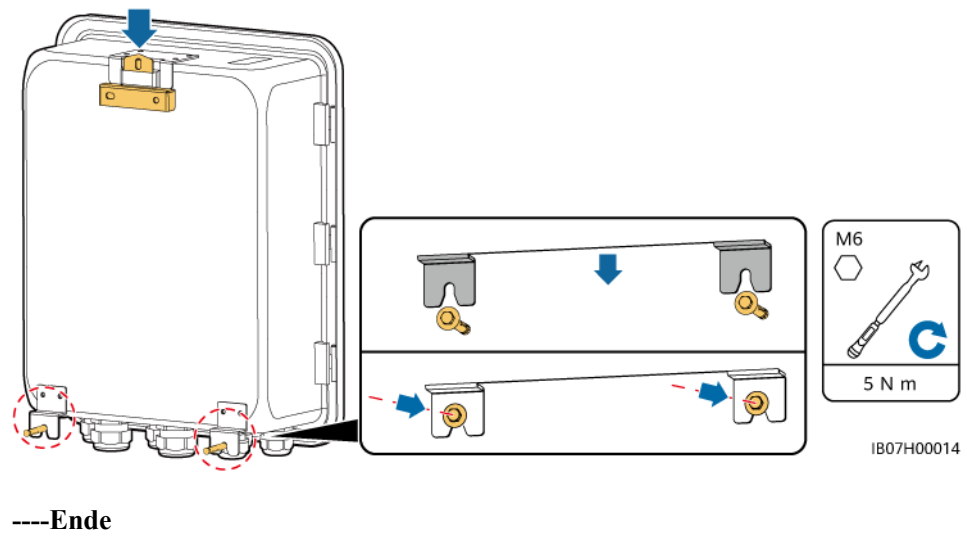
Abbildung 4-6 Montage des SmartGuard
