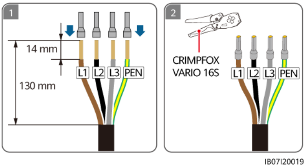
Abbildung 5-17 Crimpen der AC-Kabelendklemmen (TN-C-System)
