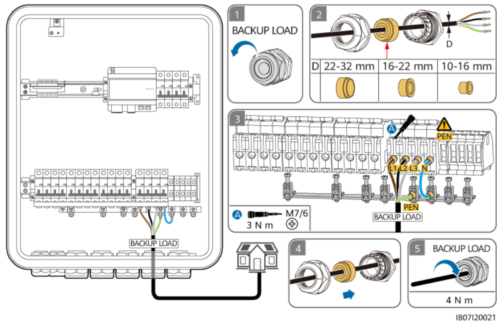
Abbildung 5-20 Anschließen des Ausgangstromkabels der Backup-Last (TN-C-System)
