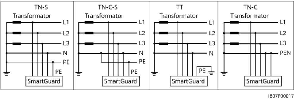
Abbildung 2-8 Erdungssysteme
