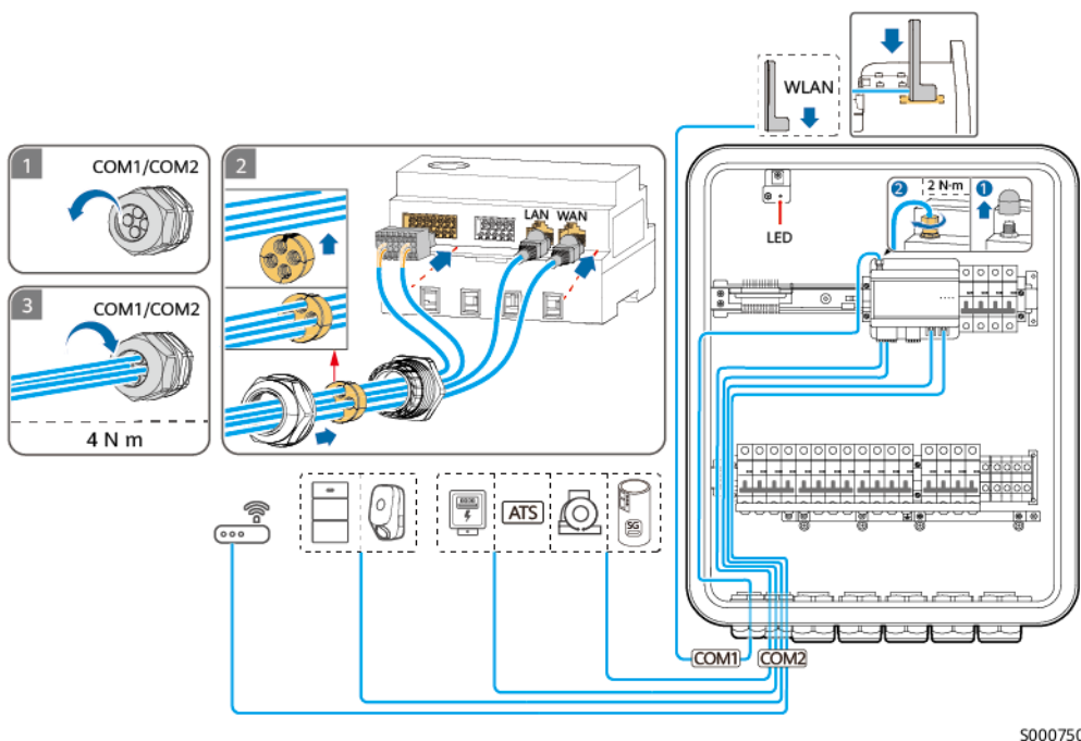
Abbildung 5-33 Anschluss von SmartAssistant-Signalkabeln (gestrichelte Kästchen weisen auf optionale Komponenten hin)
