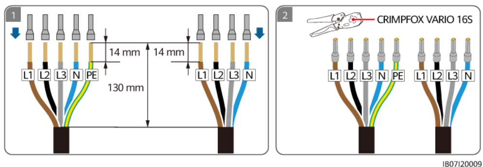
Abbildung 5-21 Crimpen der AC-Kabelendklemmen
