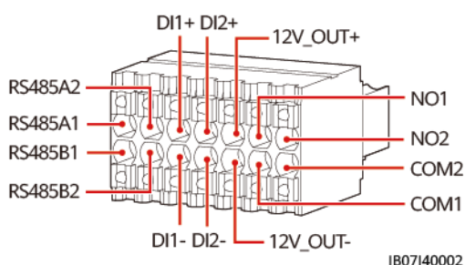
Abbildung 5-29 Pin-Definitionen
