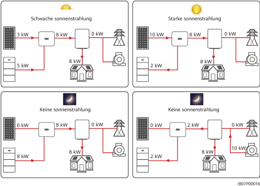
Abbildung 2-7 Darstellung der maximalen Leistung im netzentkoppelten Modus
