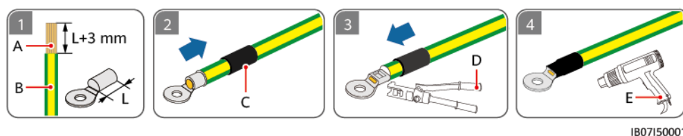
Abbildung 5-3 Crimpen eines Kabelschuhs
