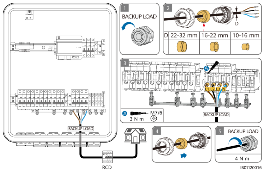
Abbildung 5-19 Anschließen des Ausgangsstromkabels der Backup-Last vom SmartGuard-63A-AUT0 (TN-S/TN-C-S/TT-System)
