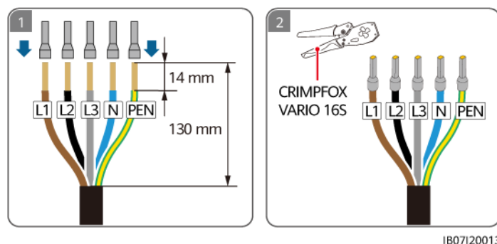
Abbildung 5-15 Crimpen der AC-Kabelendklemmen für den SmartGuard-63A-T0 (TN-S/TN-C-S/TT-System)
