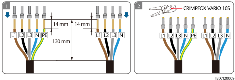
Abbildung 5-8 Crimpen der AC-Kabelndklemmen (TN-S/TN-C-S/TT-System)
