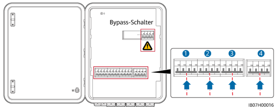
Abbildung 6-7 Einschalten der Schalter
