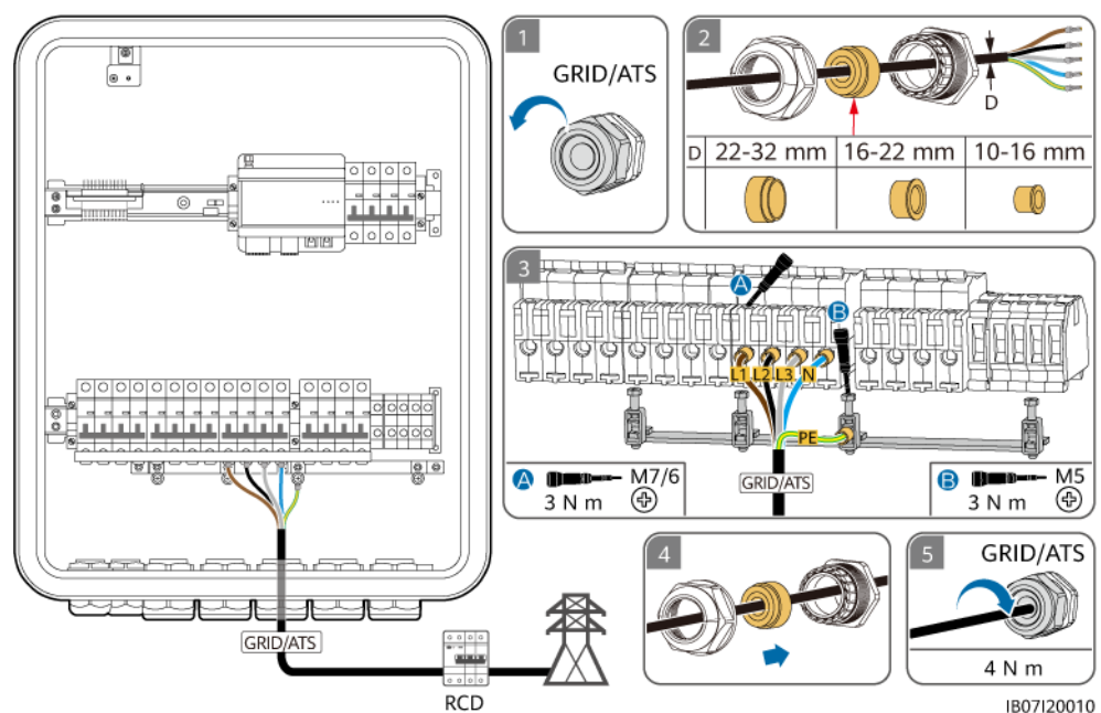
Abbildung 5-10 Anschließen des Netz-AC-Ausgangsstromkabels (TN-S/TN-C-S/TT-System)
