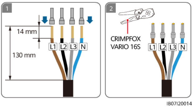
Abbildung 5-16 Crimpen der AC-Kabelendklemmen für den SmartGuard-63A-AUT0 (TN-S/TN-C-S/TT-System)
