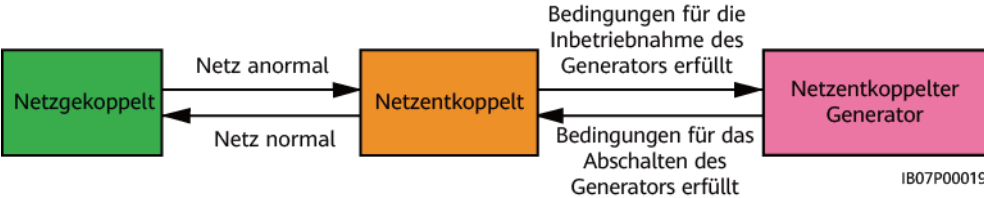
Abbildung 2-12 Arbeitsmodi
