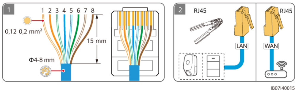
Abbildung 5-32 FE-Kommunikationskabel (gestrichelte Kästchen weisen auf optionale Komponenten hin)
