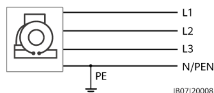
Abbildung 5-7 Generator-Nullleiter-Erdung
