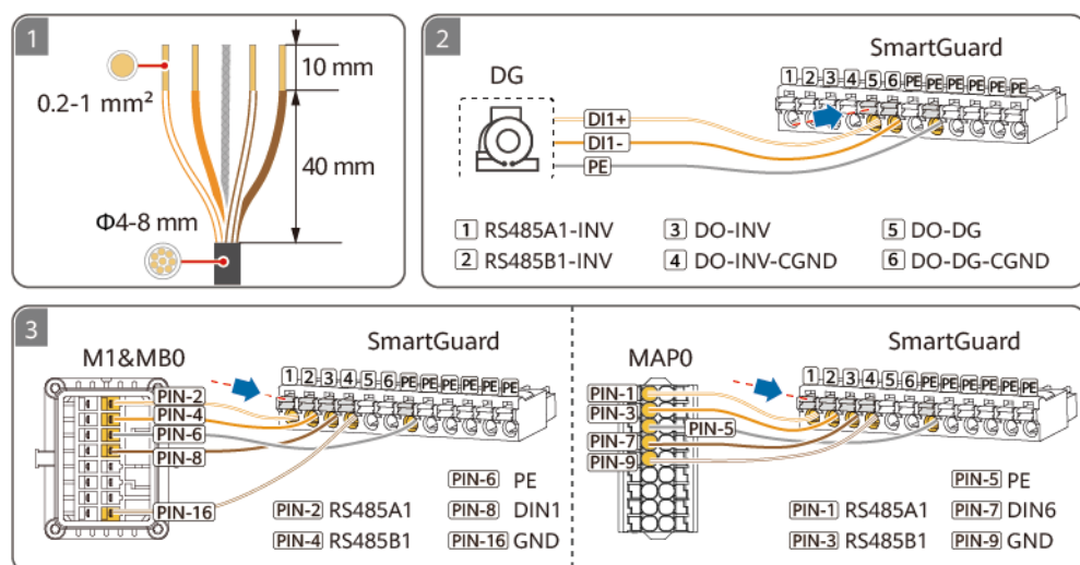
Abbildung 5-25 Crimpkabelendverschlüsse für das Signalkabel (das gestrichelte Kästchen zeigt eine optionale Komponente an)
