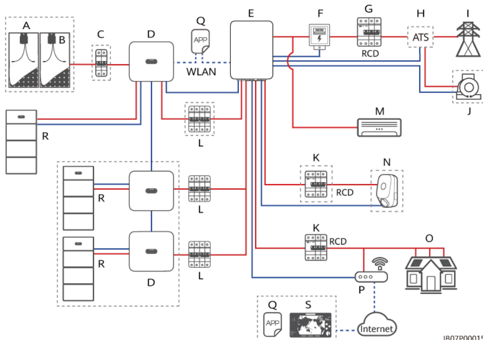
Abbildung 2-6 Vernetzung einiger Lasten, die an die SmartGuard angeschlossen sind (gestrichelte Kästchen weisen auf optionale Komponenten hin)
