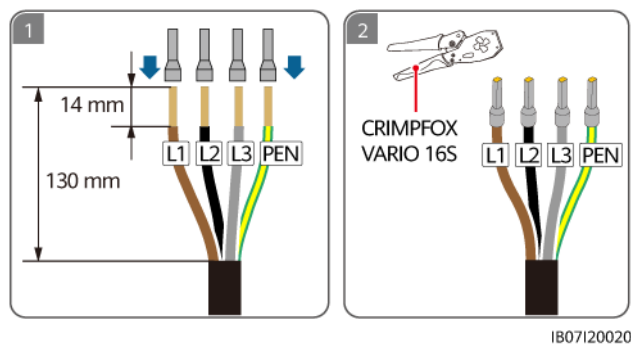
Abbildung 5-9 Crimpen der AC-Kabelndklemmen (TN-C-System)
