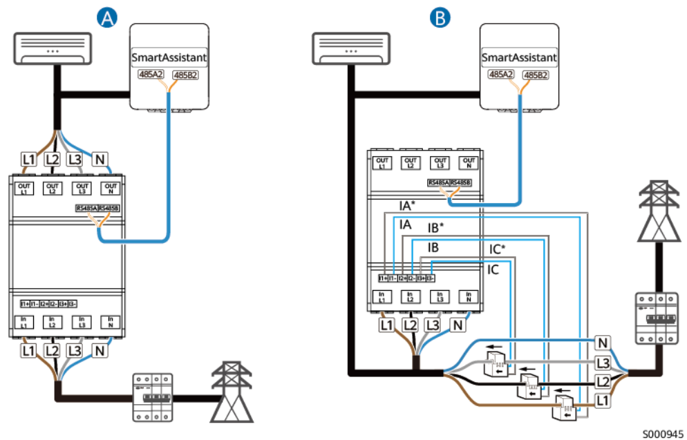
Abbildung 5-31 Anschließen des Kommunikationskabels des Stromzählers
