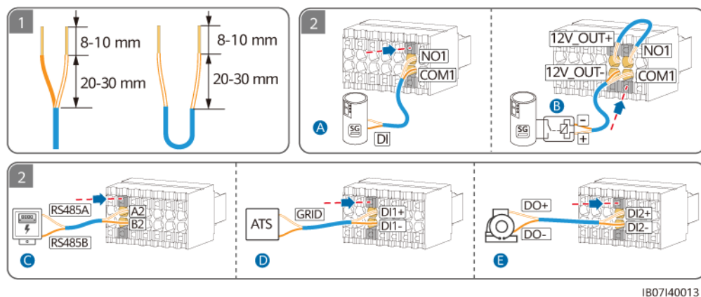
Abbildung 5-30 Anschluss des Signalkabels an die 14-polige Klemme
