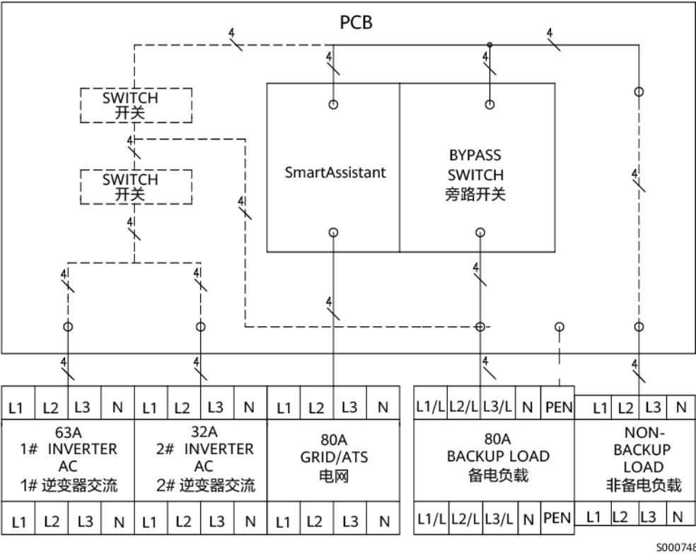
Abbildung 2-11 Elektrischer Schaltplan der SmartGuard
