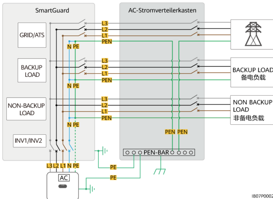
Abbildung 2-4 Schaltpläne für Eigenheime für das TN-C-System (gestrichelte Linien zeigen optionale Kabelverbindungen an)
