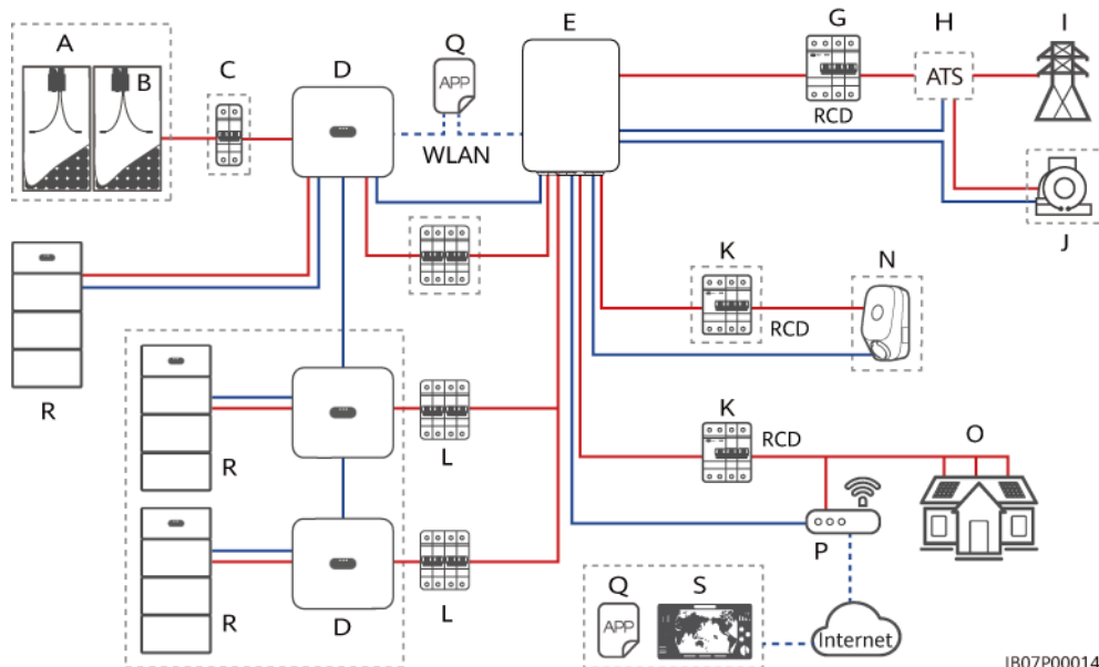
Abbildung 2-5 Vernetzung aller Lasten, die an die SmartGuard angeschlossen sind (gestrichelte Kästchen weisen auf optionale Komponenten hin)
