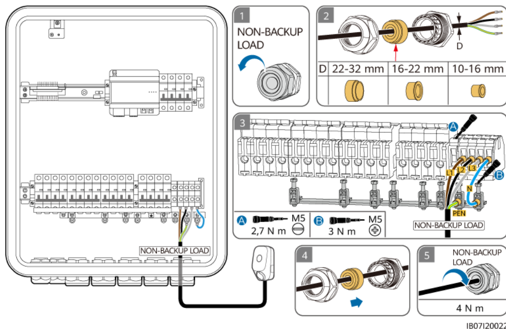
Abbildung 5-24 Anschließen des Ausgangstromkabels der Nicht-Backup-Last (TN-C-System)
