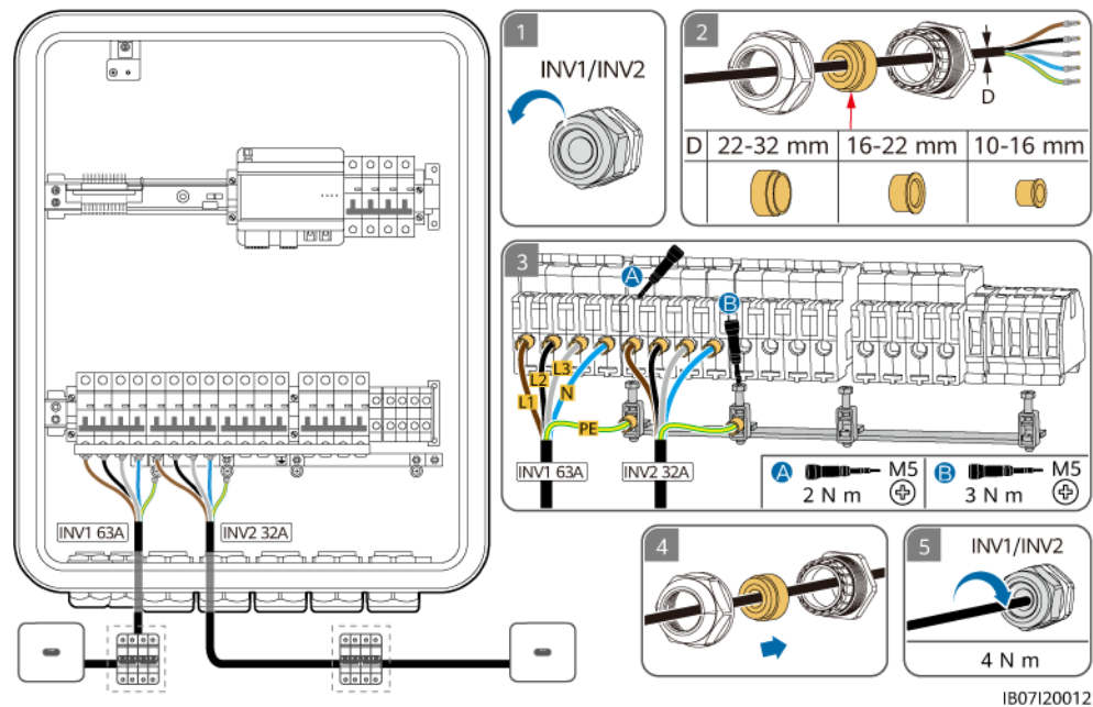
Abbildung 5-14 Anschließen der AC-Eingangsstromkabel des Wechselrichters (gestrichelte Kästchen weisen auf optionale Komponenten hin)
