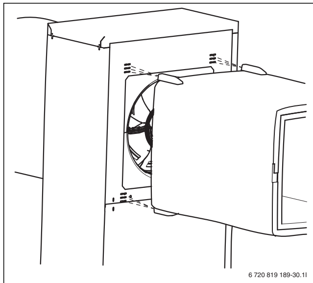
Bild 25 Luftkanal an der Luftöffnung positionieren
