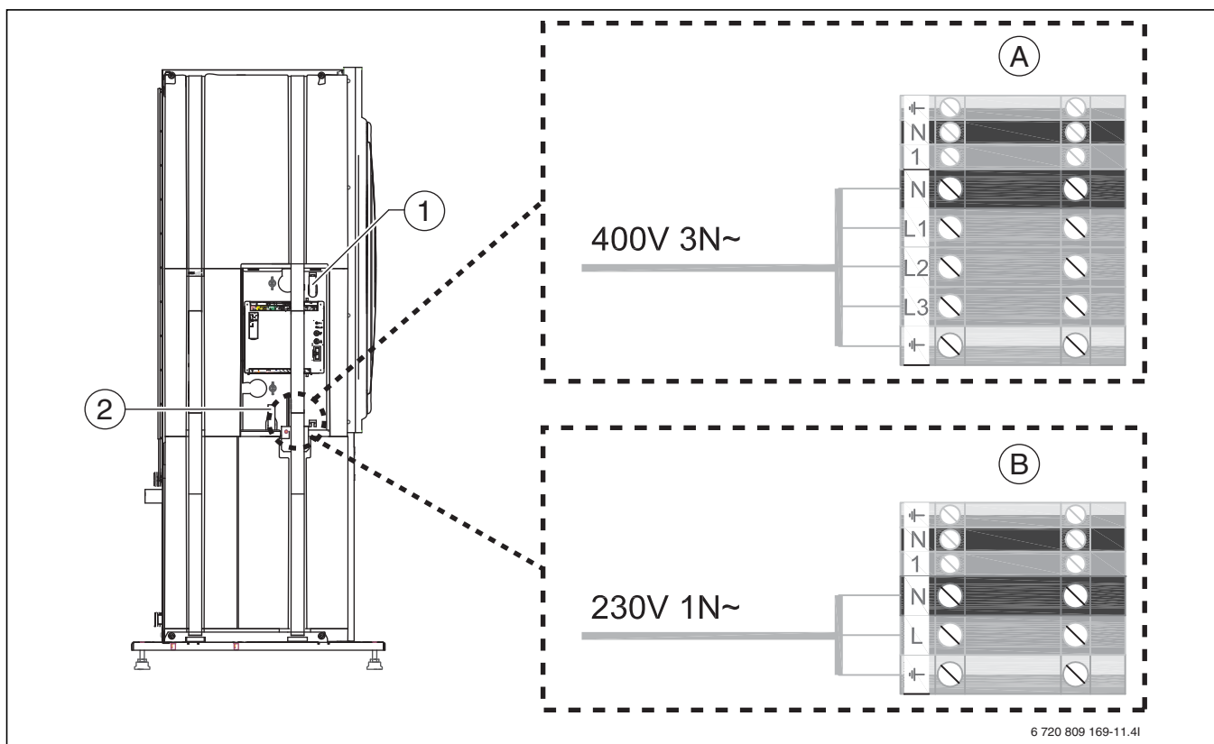
Bild 37 Kabelkanäle am Anschlusskasten der Wärmepumpe
