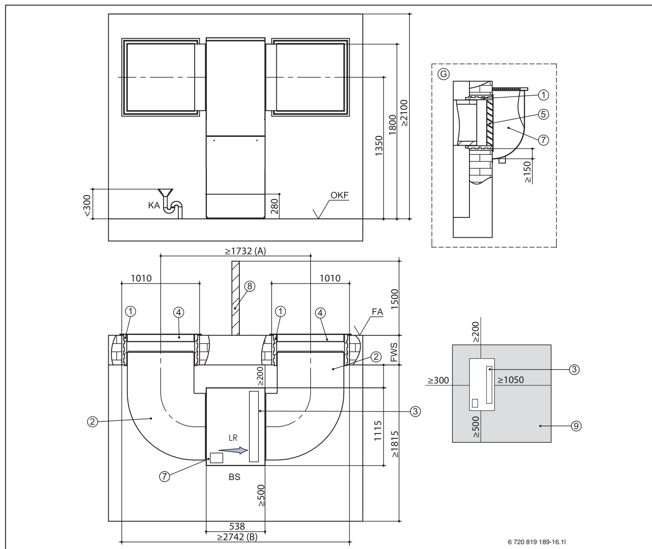
Bild 45 Kanalpläne für Luftkanalsystem für WLW196 iIR 11-14
