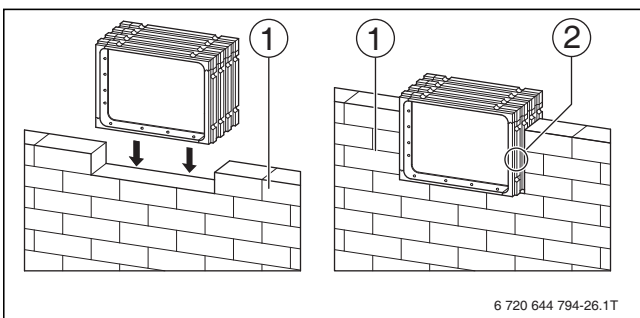
Bild 21 Wanddurchführung durch Einmauern einsetzen
