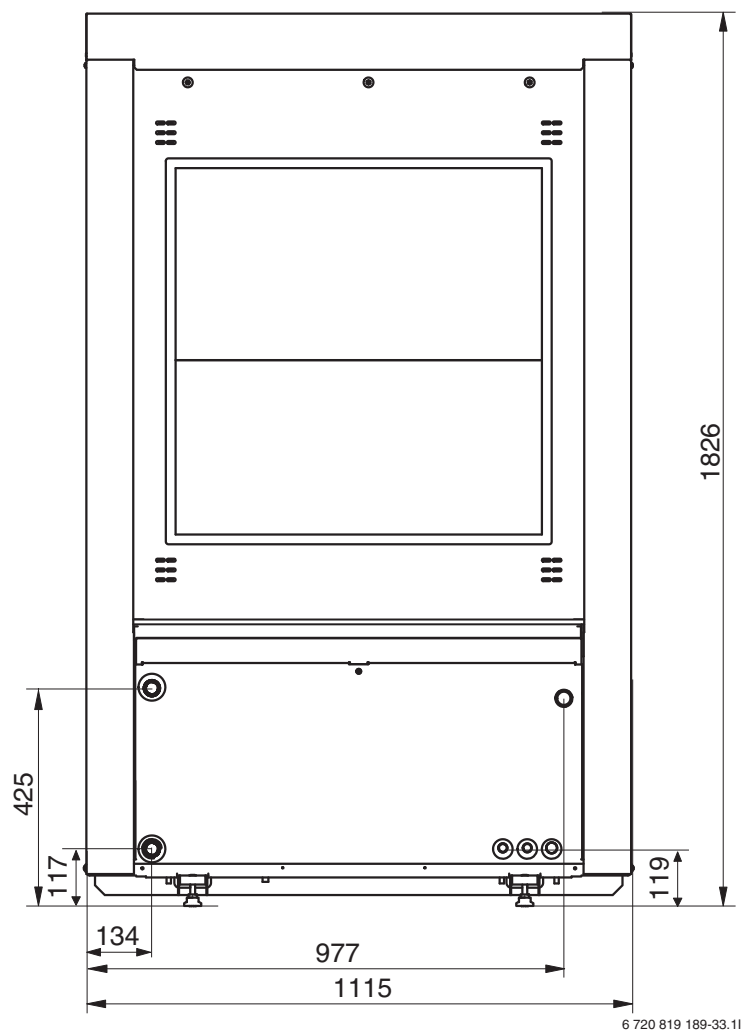
Bild 7 Abmessungen und Anschlüsse der Wärmepumpenmodelle 11–14, Rückseite
