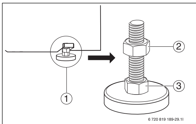
Bild 14 Standfüße montieren
