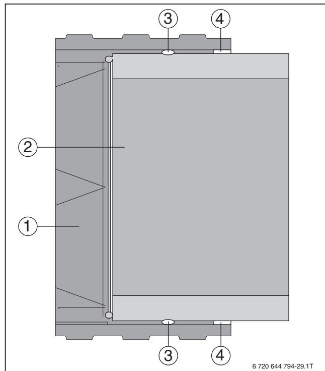
Bild 24 Luftkanal in die Wanddurchführung schieben
