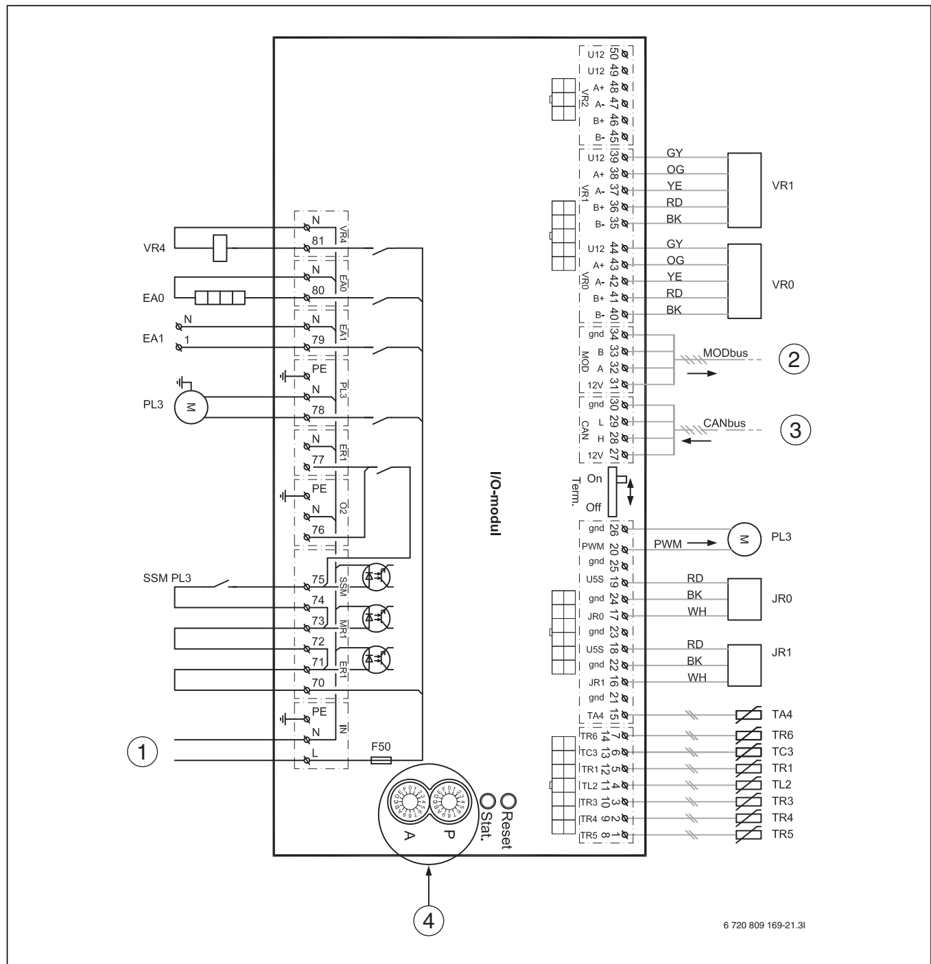
Bild 39 Schaltplan für I/O-Modulkarte
