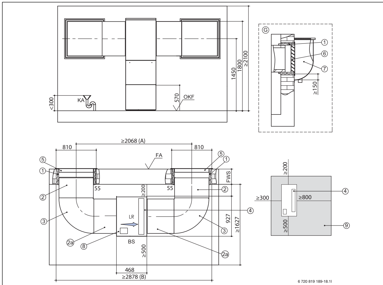
Bild 42 Kanalpläne für Luftkanalsystem für WLW196 iIR 6-8
