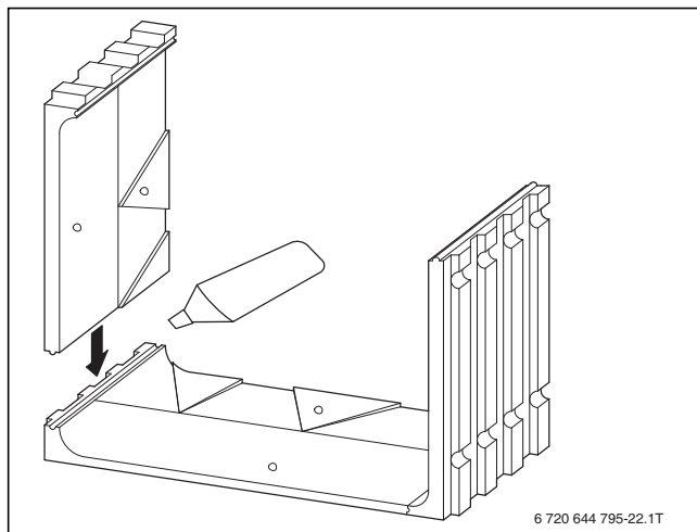
Bild 17 Weiteres Steckelement anstecken
