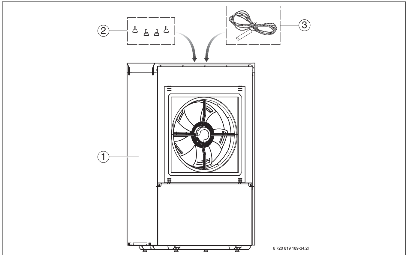
Bild 1 Lieferumfang
