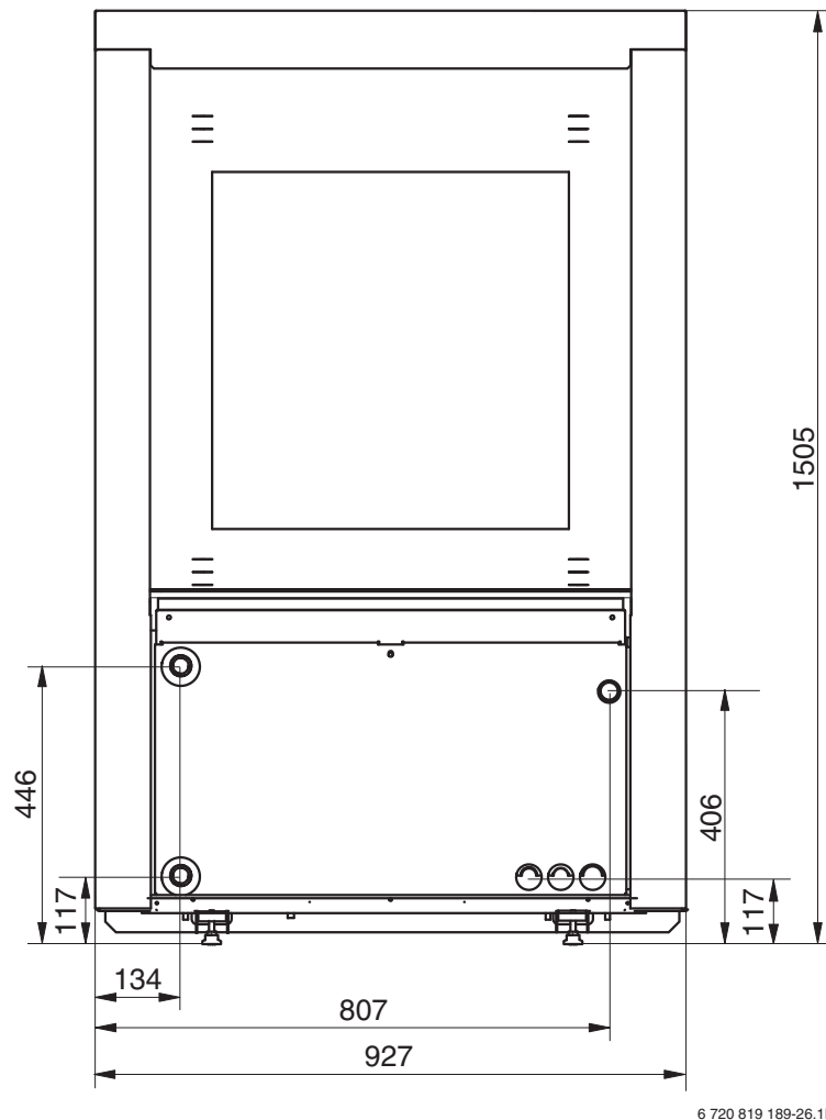
Bild 5 Abmessungen und Anschlüsse der Wärmepumpenmodelle 6–8, Rückseite
