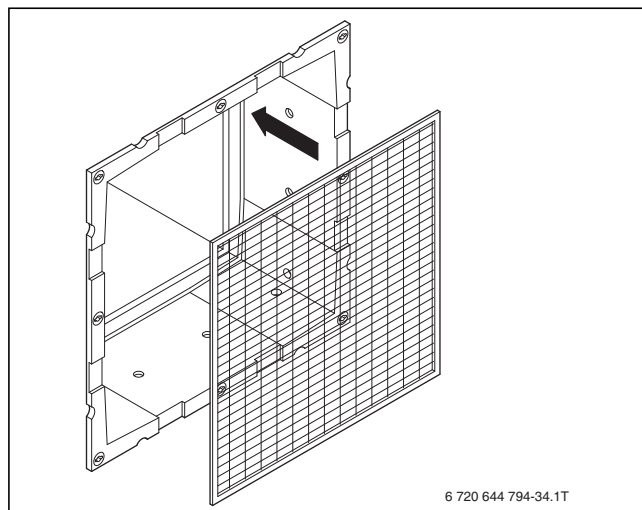
Bild 29 Maschendrahtgitter befestigen
