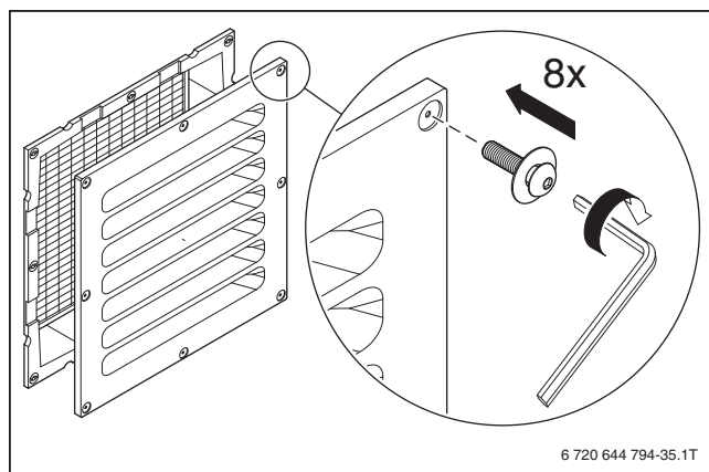
Bild 30 Wetterschutz-/Regenschutzgitter befestigen
