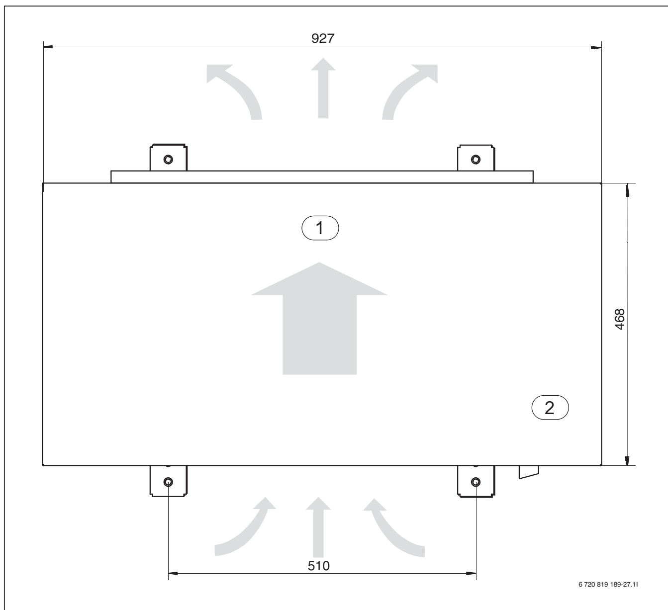
Bild 6 Abmessungen der Wärmepumpenmodelle 6–8, Draufsicht
