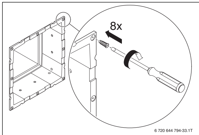
Bild 28 Einbaurahmen befestigen
