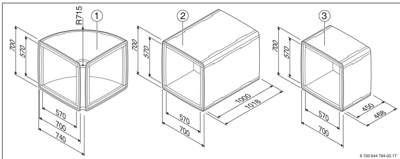
Bild 10 Luftkanäle des Systems Luftkanal 700 (alle Maße in mm)
