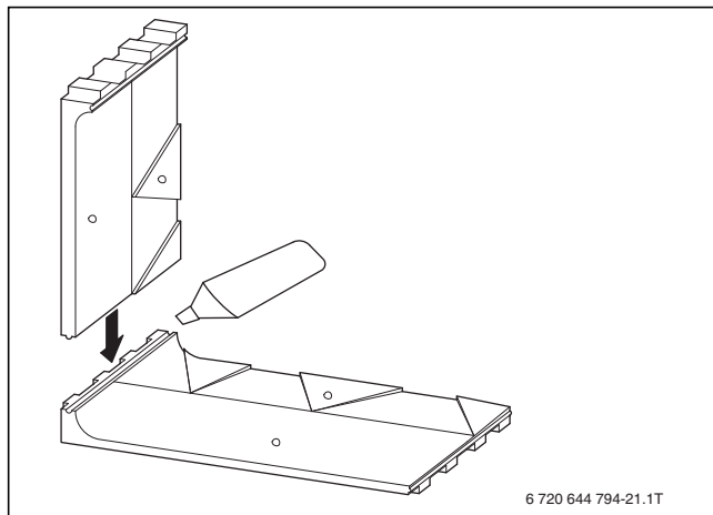
Bild 16 Steckelemente zusammenstecken
