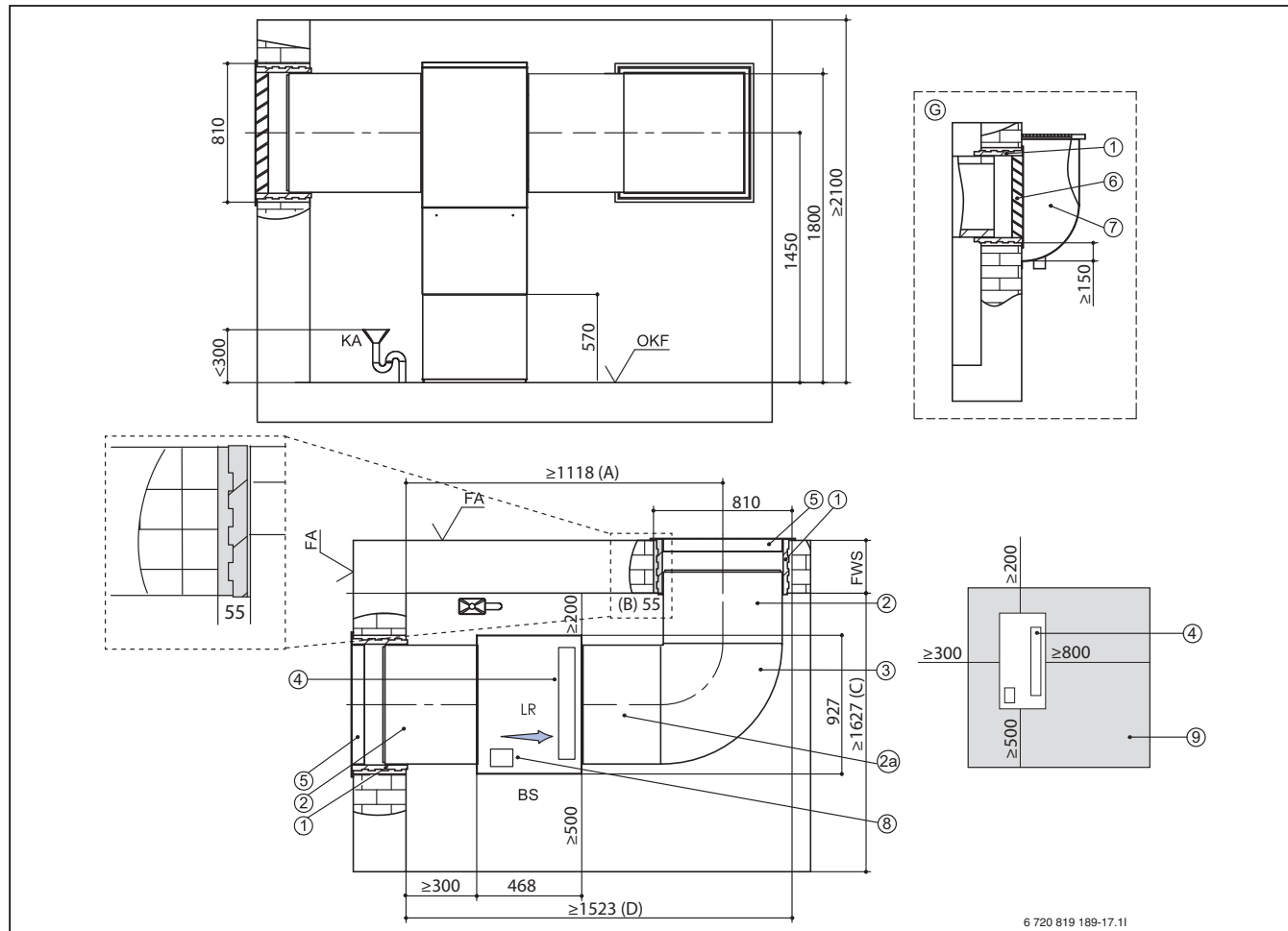
Bild 40 Kanalpläne für Luftkanalsystem für WLW196 iIR 6-8
