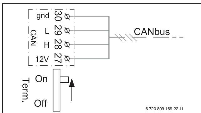
Bild 34 CAN-BUS-Terminierung
