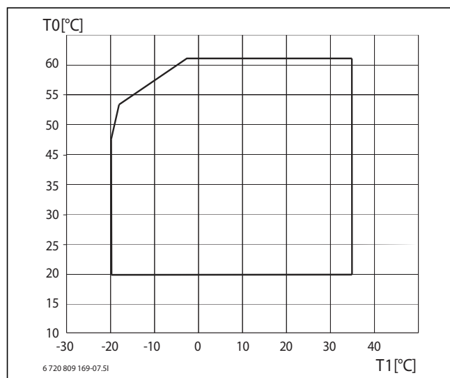
Bild 2 Wärmepumpe ohne Zuheizung
