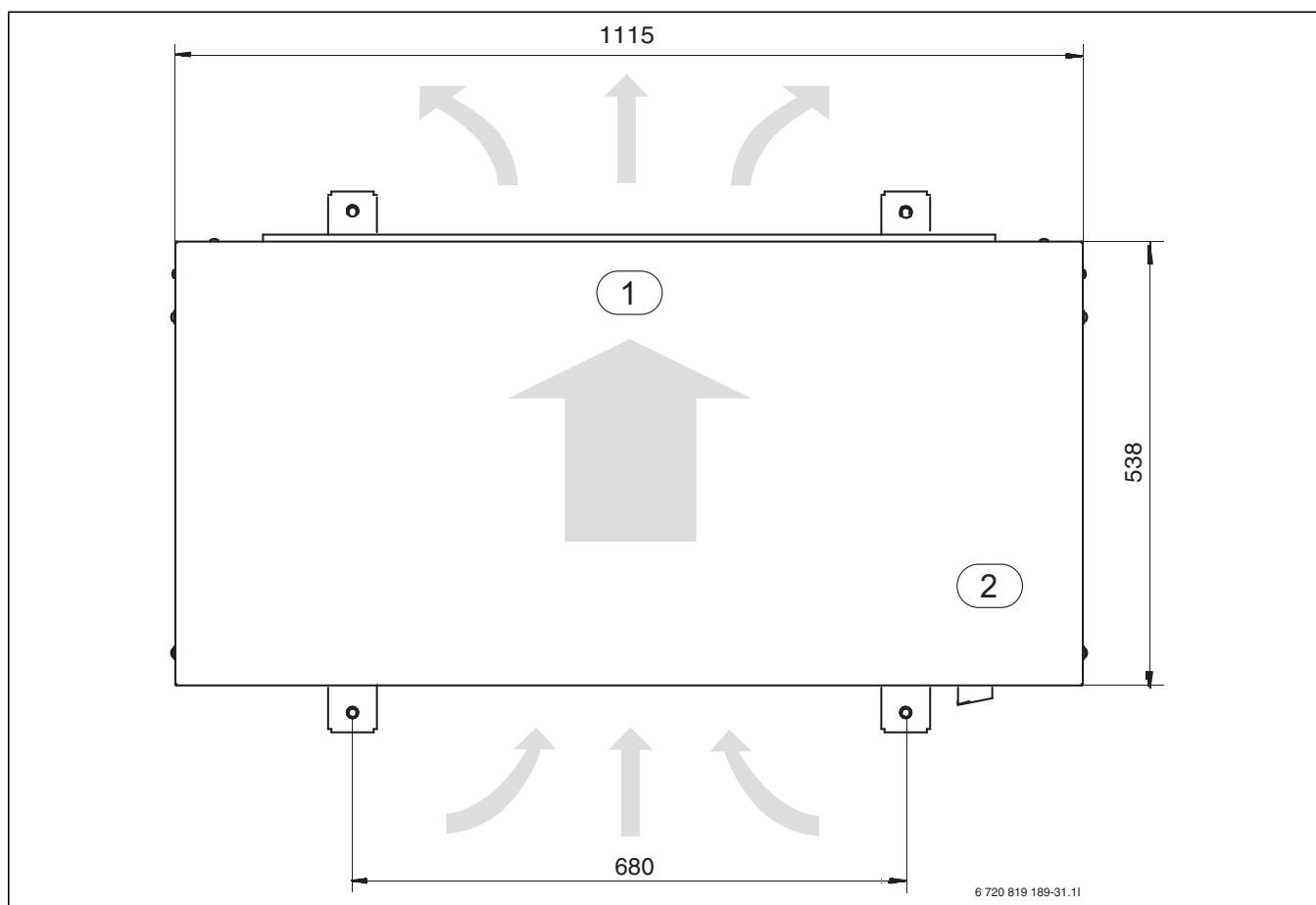
Bild 8 Abmessungen der Wärmepumpenmodelle 11–14, Draufsicht
