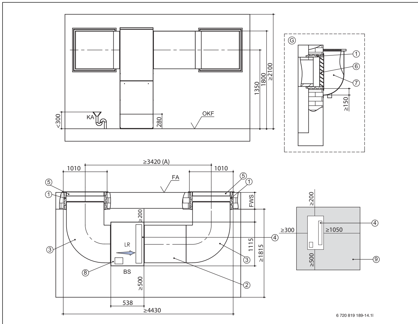
Bild 44 Kanalpläne für Luftkanalsystem für WLW196 iIR 11-14
