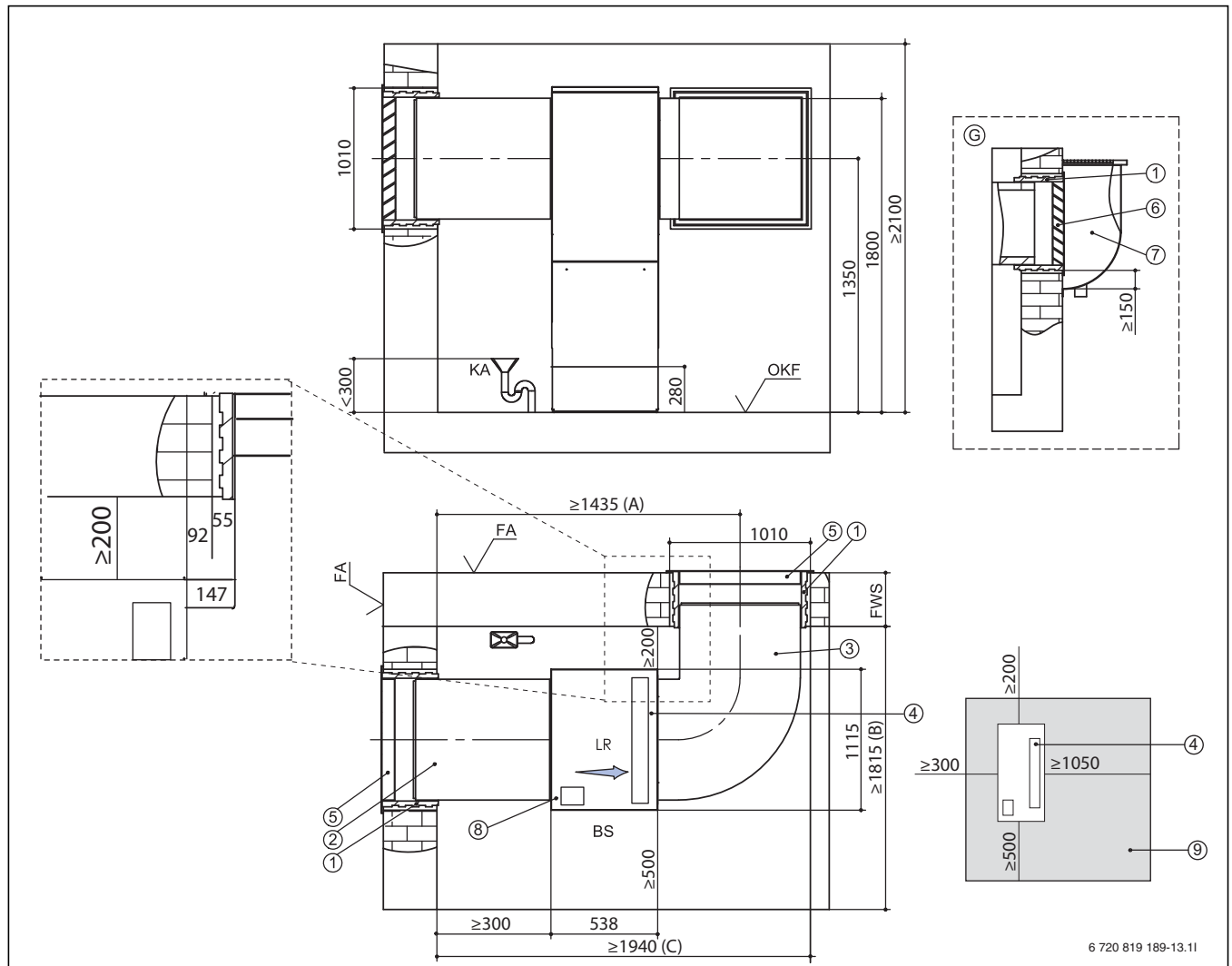
Bild 43 Kanalpläne für Luftkanalsystem für WLW196 iIR 11-14
