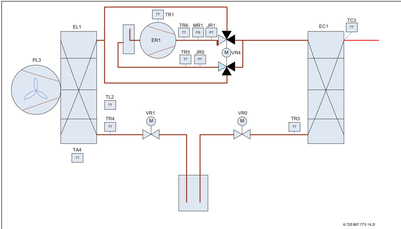
Bild 3 Kältekreis
