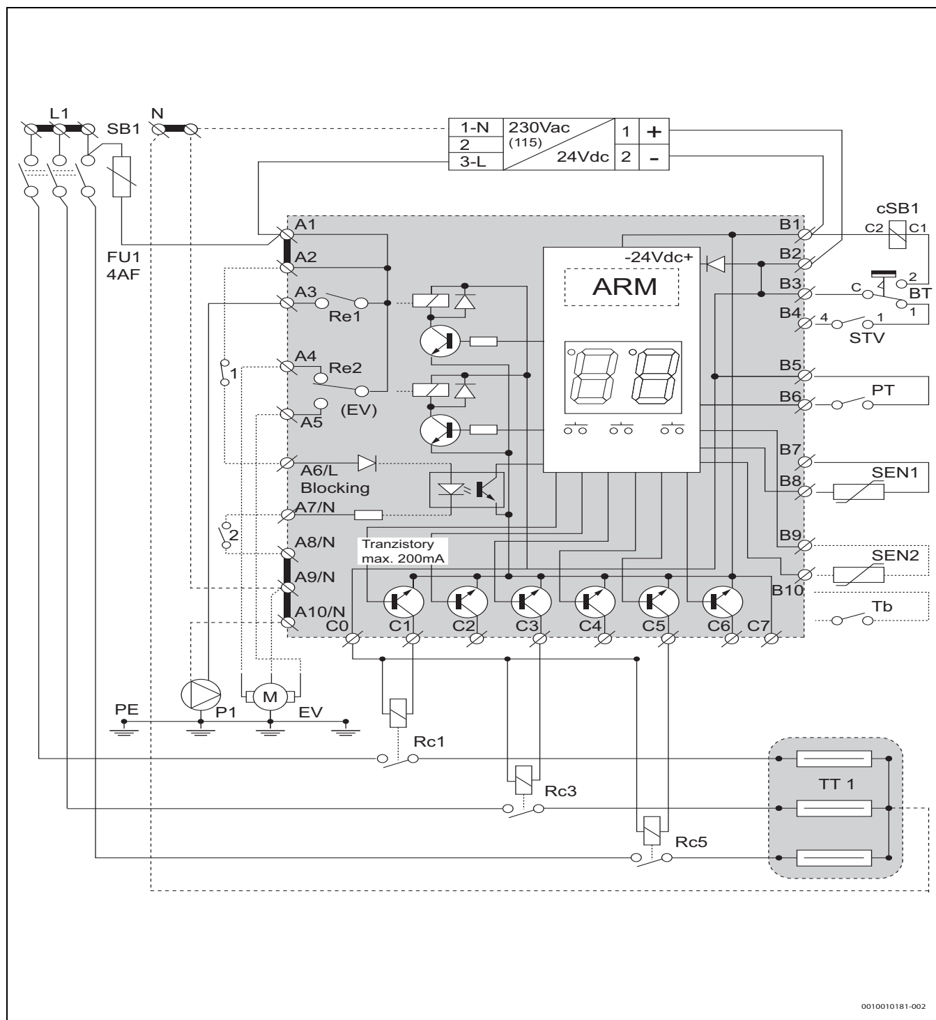
Bild 19 Anschlussplan des Heizgeräts Logamax E156 (4-12 kW), 1x 230 V AC
