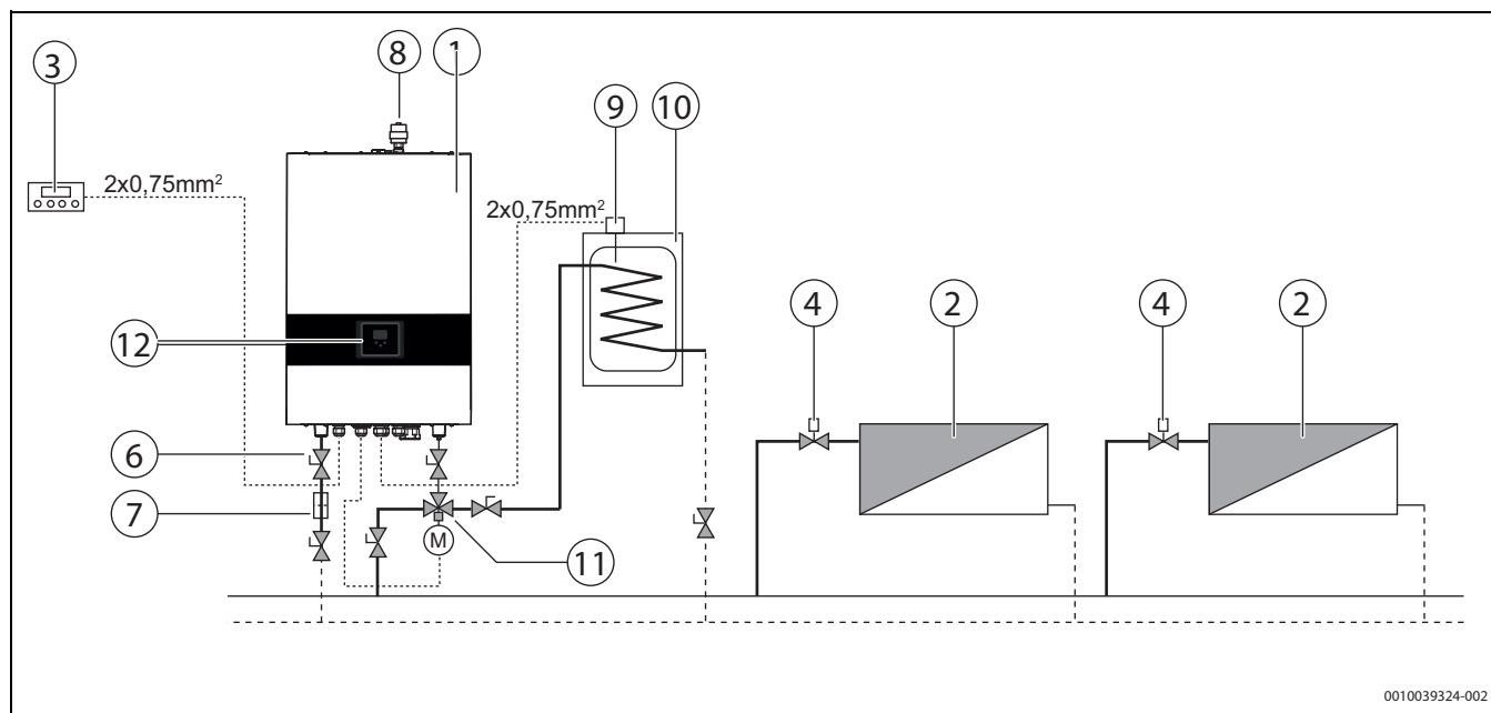
Bild 40 Heizbetrieb und WW-Bereitung mit Warmwasserspeicher
