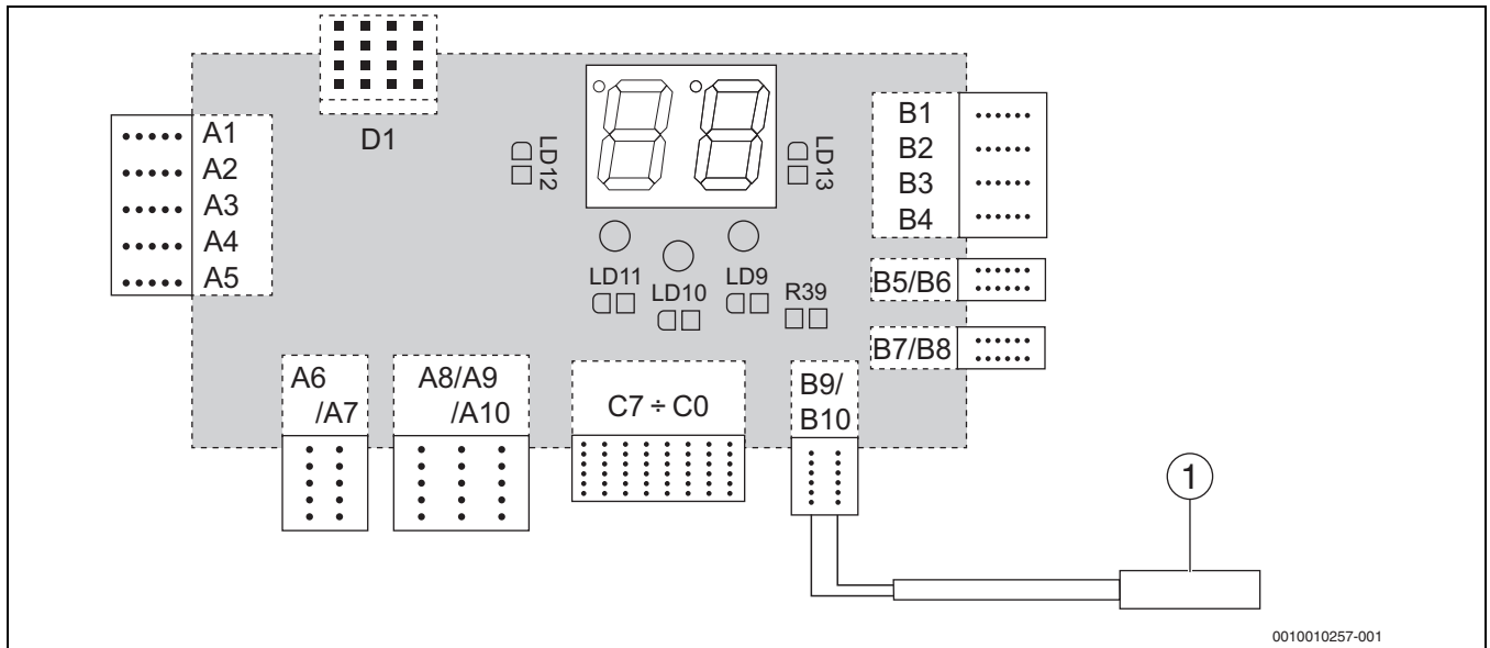
Bild 32 Anschluss eines externen Temperatursensors für die minimale Raumtemperatur oder eines zusätzlichen Raumthermostats
