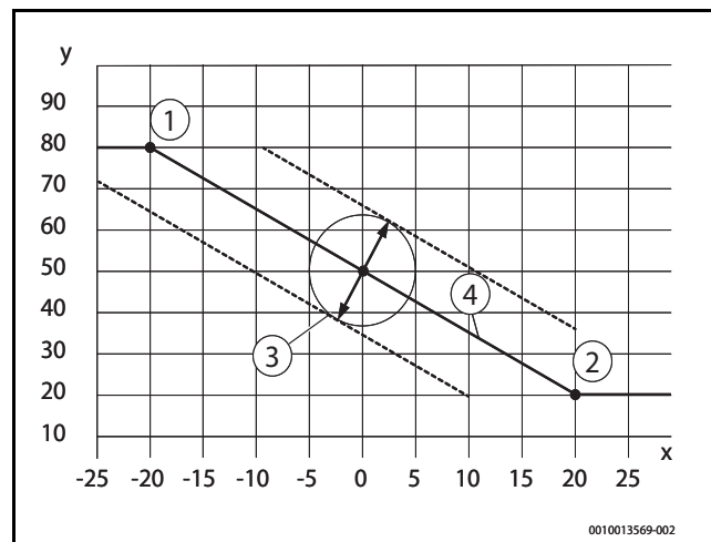
Bild 35 Außentemperaturgeführte Heizkurve
