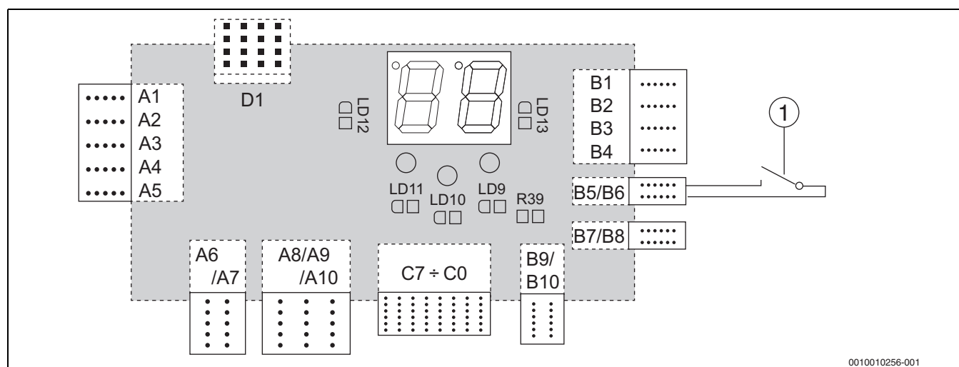
Bild 23 Anschluss Raumthermostat
