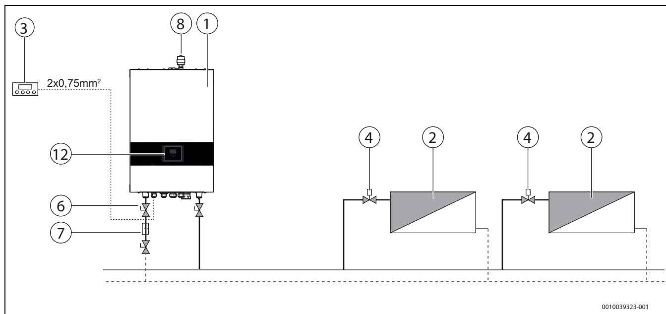
Bild 39 Nur Heizbetrieb
