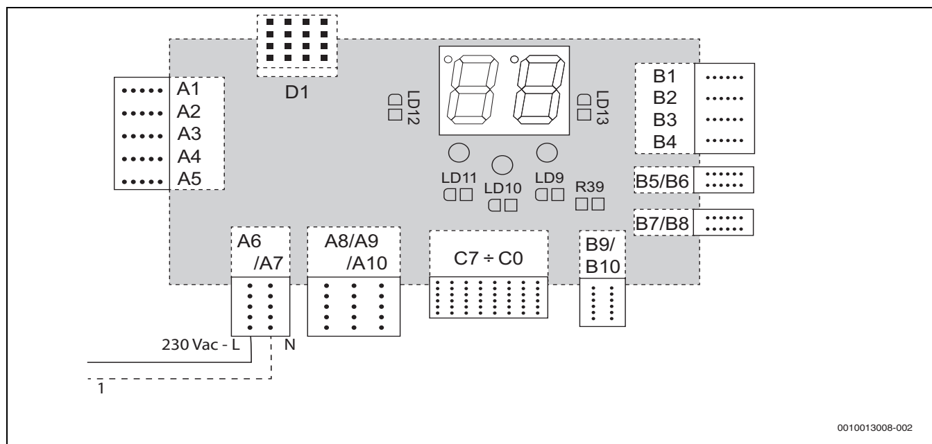
Bild 28 Steuerung des Heizgeräts durch Fernsteuerung (externe Spannung)
