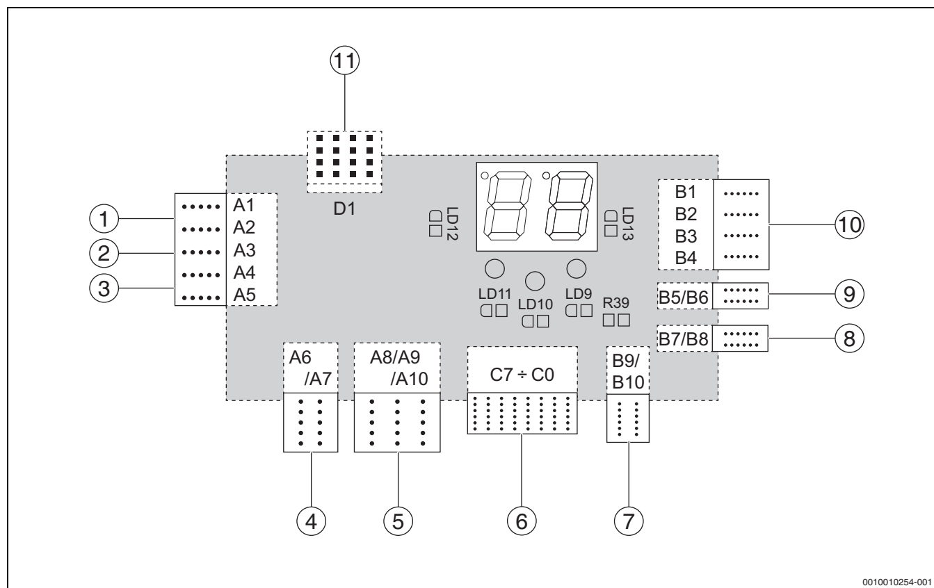
Bild 22 Elektronik Heizgerät
