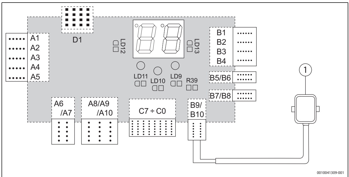
Bild 33 Anschluss eines Außentemperatursensors für die außentemperaturgeführte Regelung
