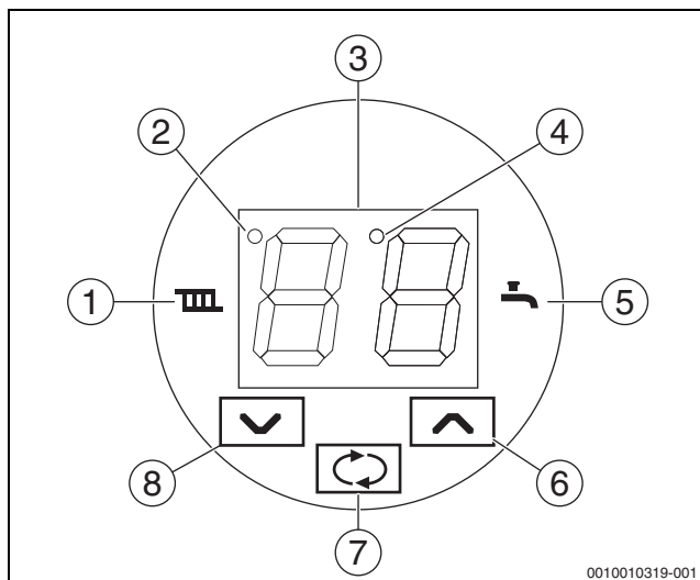
Bild 34 Bedienfeld
