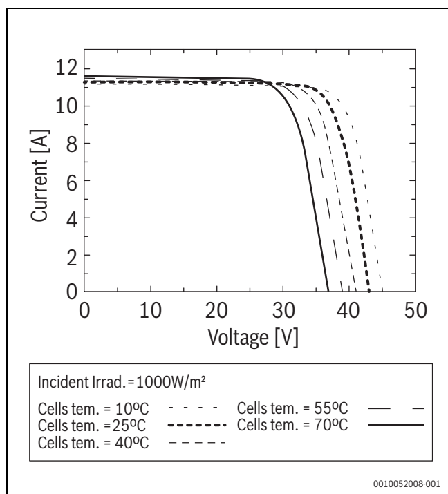
Bild 14 I-V-Kennlinie des Moduls bei unterschiedlicher Bestrahlungsstärke
