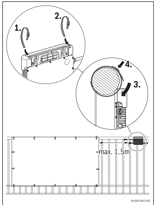
Bild 6 Installation des Mikrowechselrichters am Geländer
