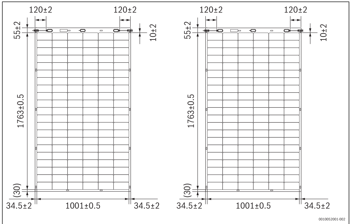
Bild 2 Abmessungen des Moduls (mm)
