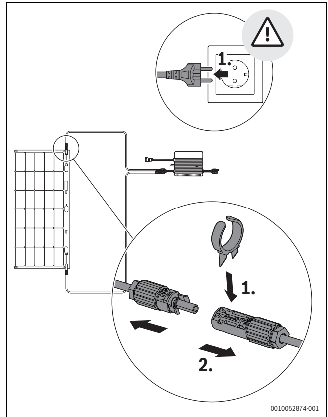
Bild 12 Steckverbinder des DC-Kabels trennen
