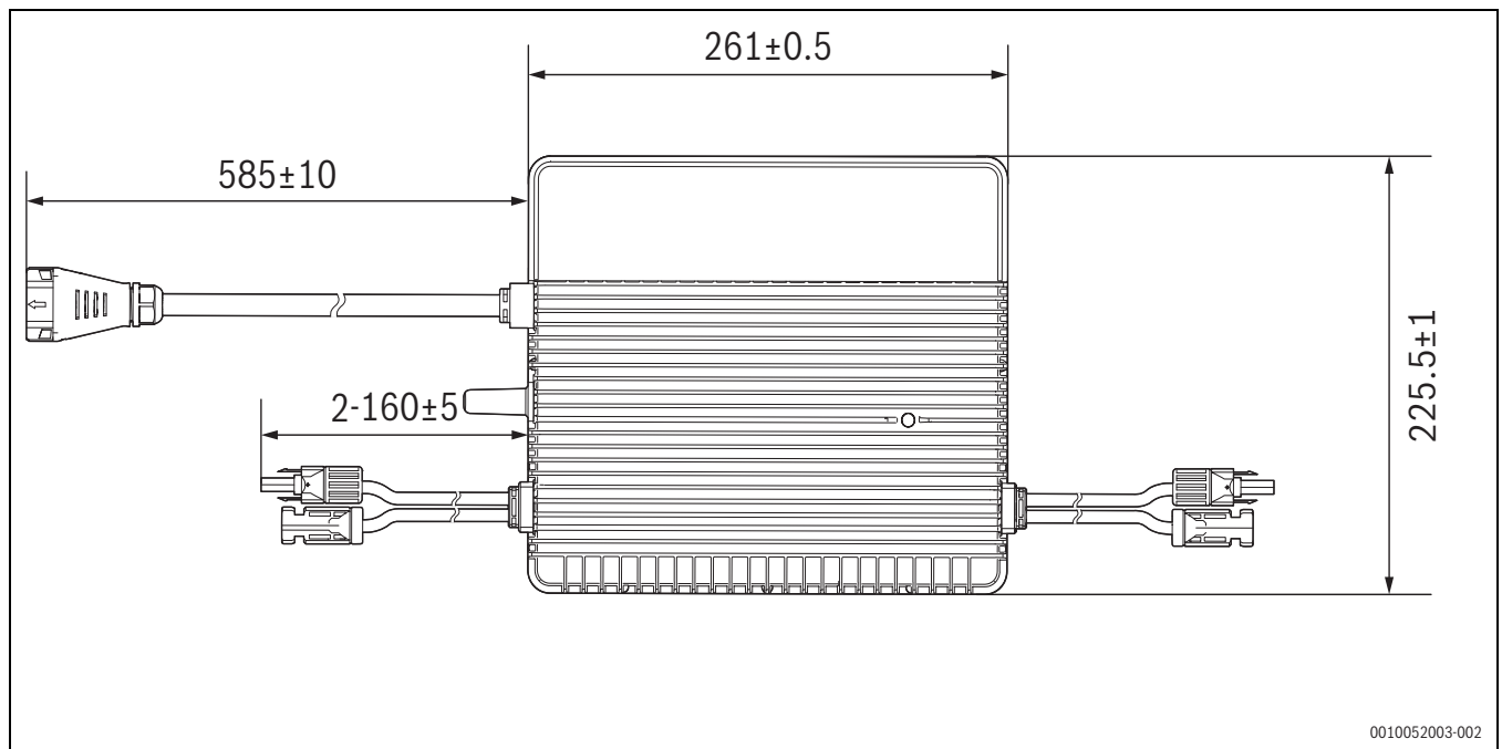
Bild 3 Abmessungen des Mikrowechselrichters (mm)
