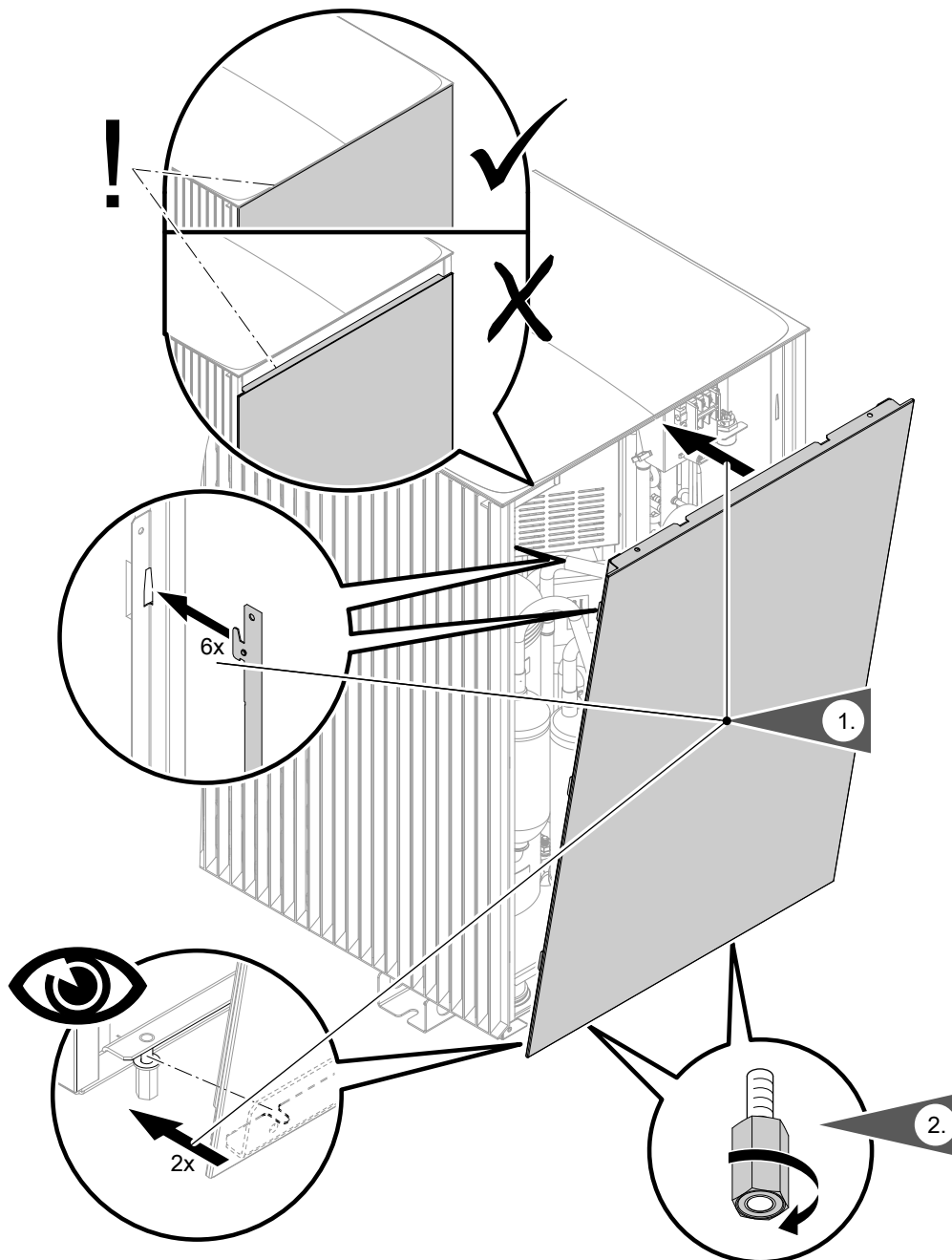
Anzugsdrehmoment 5,0 +1,0 Nm
